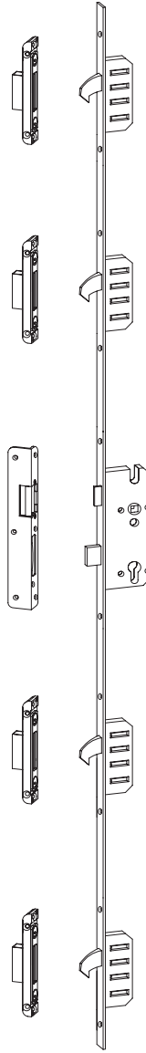
M4 4개 후크가 있는 5중 잠금장치 색상: top zinc
